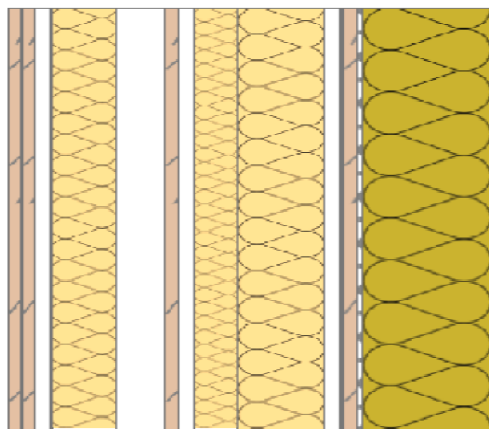
Stratigrafia di muratura esterna con sistema a secco e cappotto
